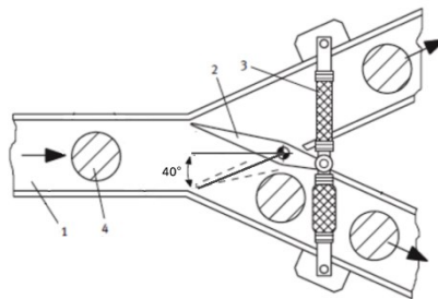
Рис. 1. Схема на основі пневмомускулів. 1 - сортувальна заслінка; 3 - об'єкти для сортування
