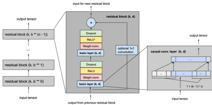
Рис. 1. Архітектура тимчасово згорткової мережі
