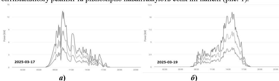
Рис.1. Fronius. Генерація за погодних умов 17.03.25 (а) і 19.03.25 (б): нижній графік - МРРТ2, середній - МРРТ1, верхній – сумарна генерація.
