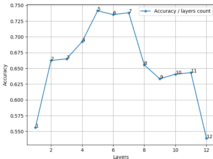
Рисунок 1. Зміна точності класифікації зі збільшенням глибини мережі.
