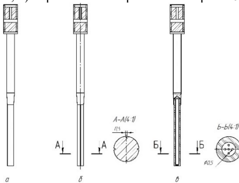
Рис. 1. Конструкції поршнів
