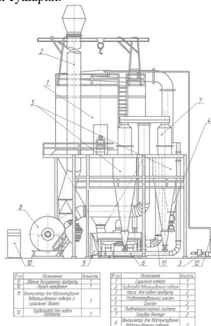
Рис. 1. Загальний вигляд сушильного комплексу для крові
