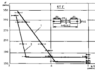
Рис. 1. Криві втоми сталі 65Г. 1 – еталонна; 2 – лазерне опромінення
