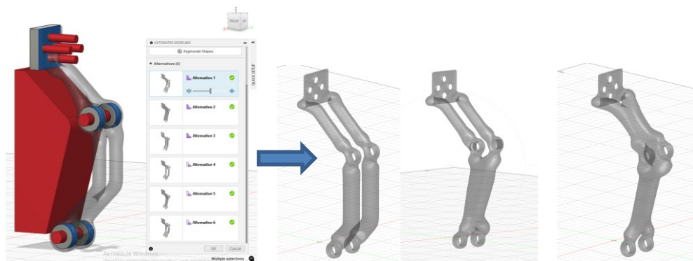
Рис. Результати моделювання конструкції захвату з використанням генеративного дизайну
