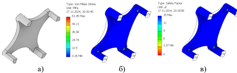
Рис. 2. Оптимізована модель платформи та результати розрахунку: а) – оптимізована 3D-модель платформи; б) – напруження по Мізесу; в) – коефіцієнт запасу міцності
