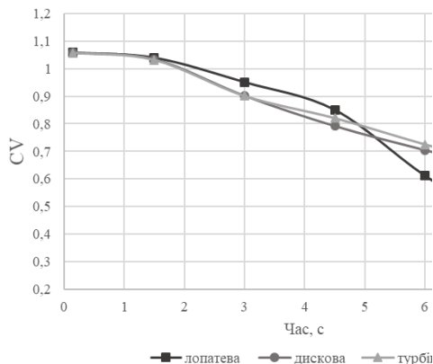
Рис.1. Коефіцієнт дисипації для різних типів перемішувачів елементів: лопатевої, дискової, турбінної
