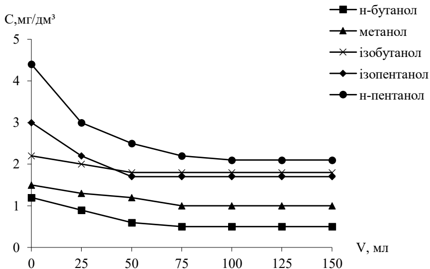
Рис. 1. Зміна покомпонентного вмісту вищих спиртів у сортівках залежно від об'єму розчину, пропущеного крізь шар глауконіта
