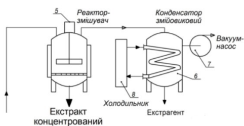
Рис. 1. Метод з використанням вакуумного реактора випарювання.
